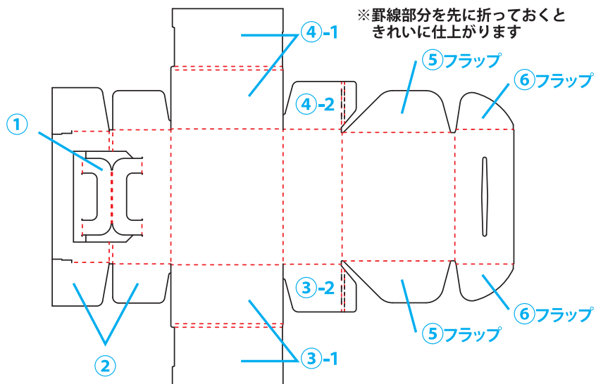
▲ 展開図
